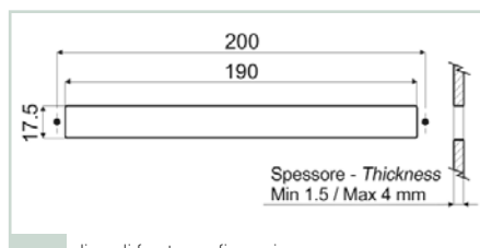
O dima di foratura e fissaggio drilling and fixing template
